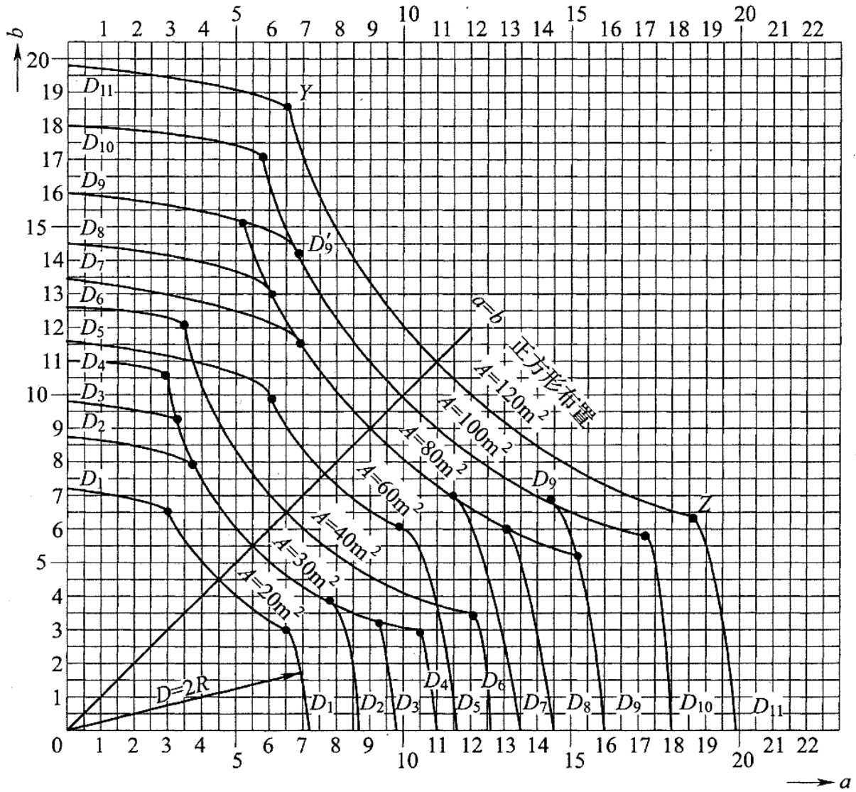
图 E 探测器安装间距的极限曲线
